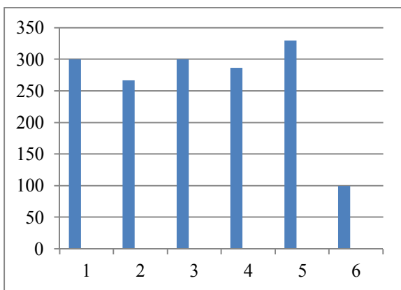
Рис.2. Величина теплового потока через стены при общепринятых толщинах, % / The heat flux through the wall in the conventional thicknesses, %
