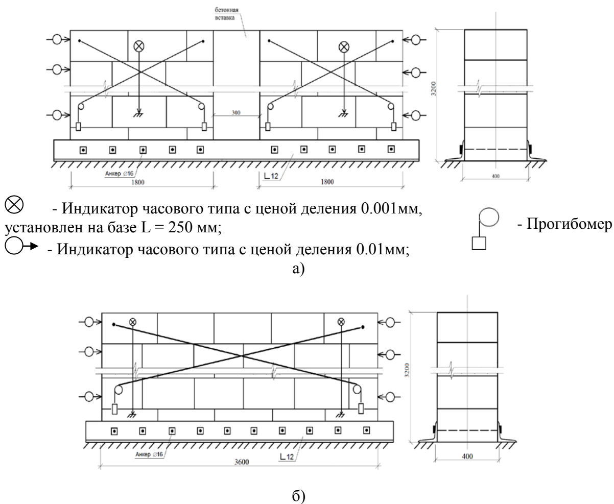
Рис. 7. Схемы установки приборов для измерения горизонтальных перемещений и перекосов фрагментов при испытании на знакопеременные сдвиговые нагрузки кладки с сердечником (а) и при его отсутствии (б)
