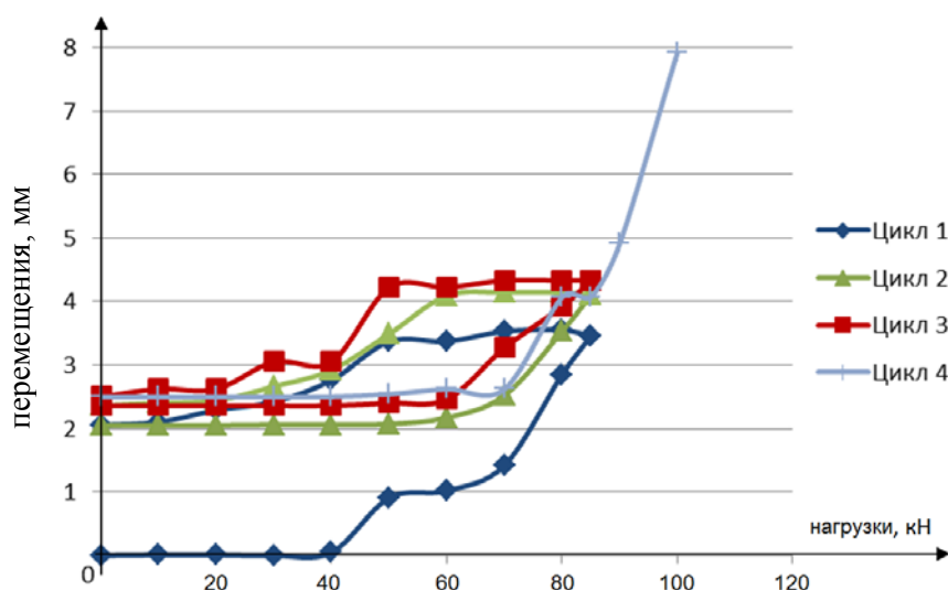
Рис. 9. Гистерезисные зависимости перемещений верха натурального простенка от горизонтальной нагрузки
