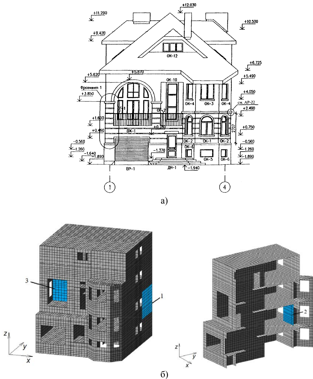
Рис. 2. Фасад жилого дома с несущими стенами из газобетонных блоков (а) и пространственная модель здания (б)
