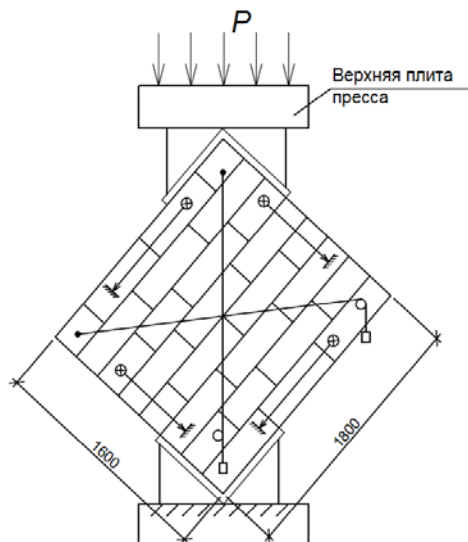
Рис. 4. Схема установки измерительных приборов при испытании фрагментов кладки на перекос
