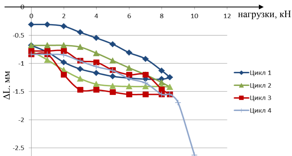
Рис. 8. Гистерезисные зависимости удлинения диагонали натурального простенка от горизонтальной нагрузки
