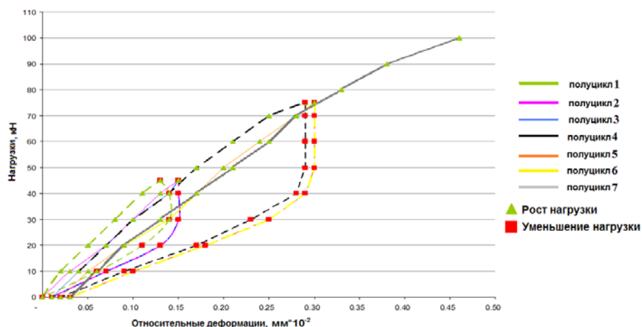
Рис. 6. Гистерезисные зависимости фрагмента ФГ-2ц
