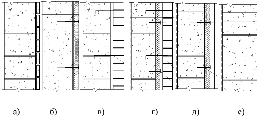
Рис. 2. Конструктивные решения и системы отделки стен из автоклавного газобетона а) облицована плиткой керамической; б) с тонкослойной системой утепления; в) облицована кирпичом с вентилируемым воздушным зазором; г) облицованная кирпичом с дополнительной теплоизоляцией; д) с «навесным вентилируемым фасадом»; е) – однослойная стена отделанная штукатуркой;
