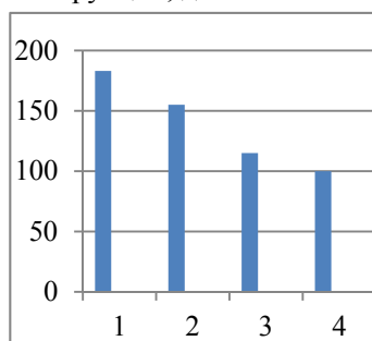
Рис. 1. Затраты на возведение стен, % 1. Кирпич керамический пустотелый с ССТ 2. Кирпич силикатный полнотелый с ССТ 3. Блоки из известняка ракушечника с ССТ 4. Автоклавный газобетон
