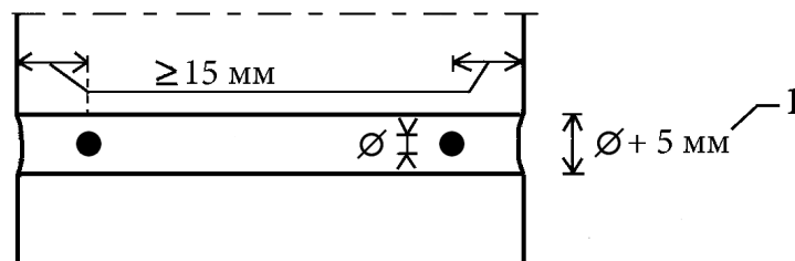
Рисунок 13.2 – Захисний шар розчину у ложкових швах кладки
