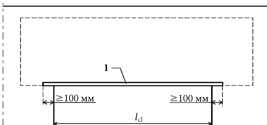
Рисунок 11.8 – Комбінована перемичка, що утворює балку-стінку
