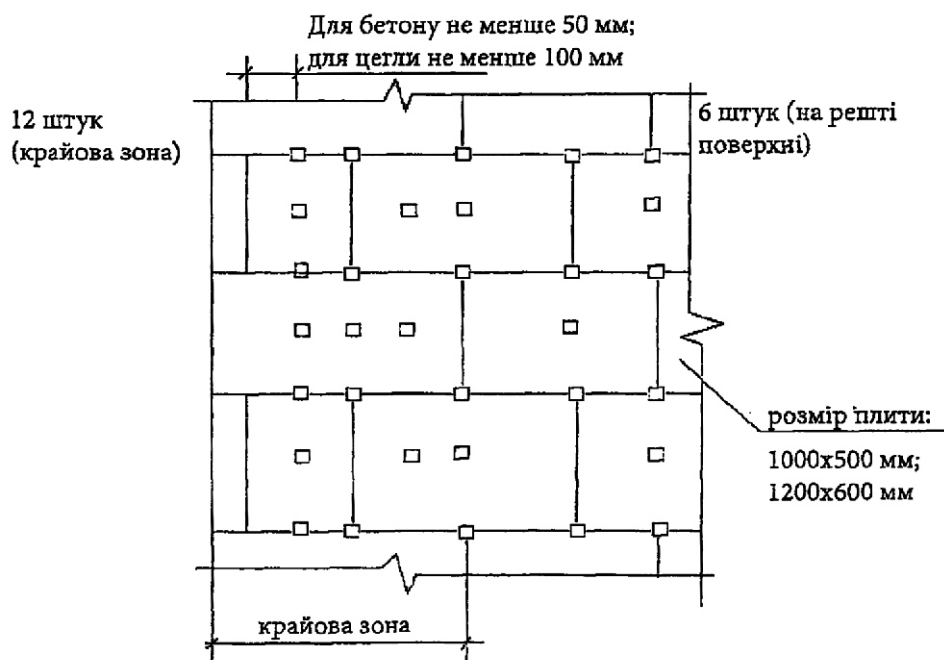
Схема розташування дюбелів у зоні по краях
