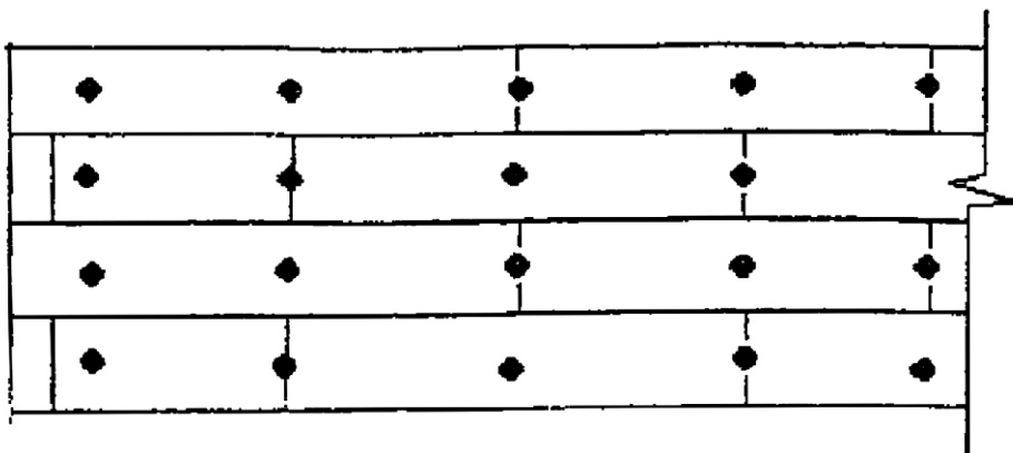
Схема розташування дюбелів у зоні по краях Розмір плити: 1200 мм 200 мм, 1200 мм 150 мм
