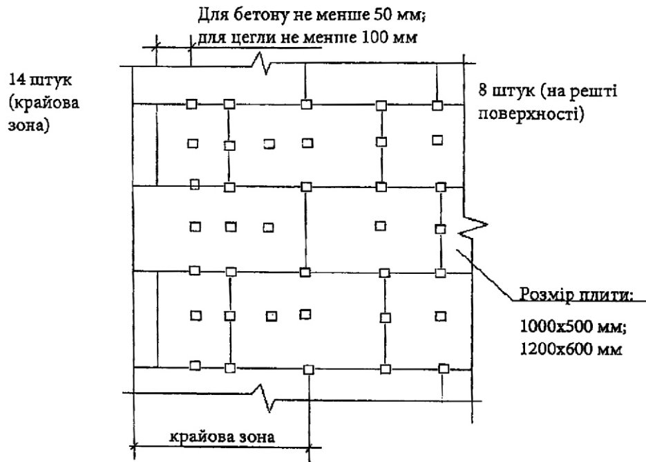
Схема розташування дюбелів у зоні по краях
