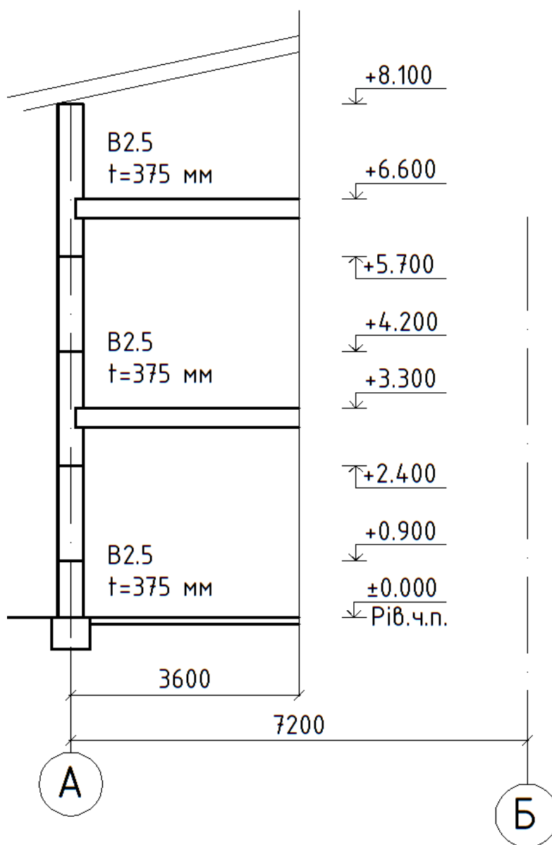
Рис.2.3-4. Результати розрахунку простінку зовнішньої стіни
