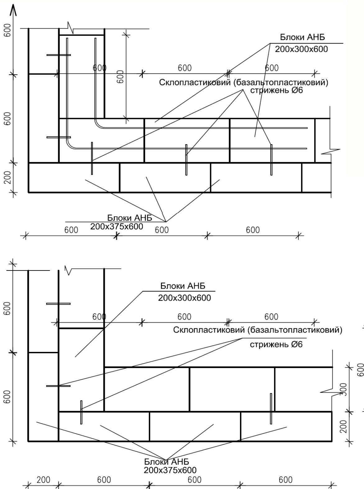
Рис.2-12-5. Двошарова стіна першого типу. Фрагмент глухої стіни. Кут кладки
