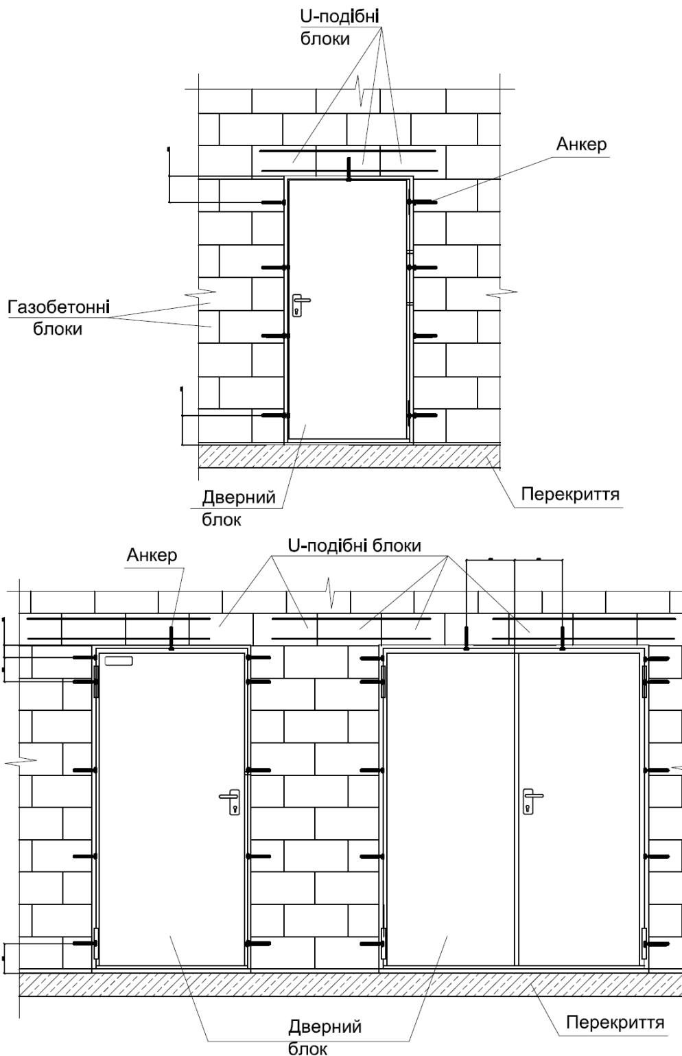
Рис.2.11-2. Схема анкерування дверей в дверних отворах
