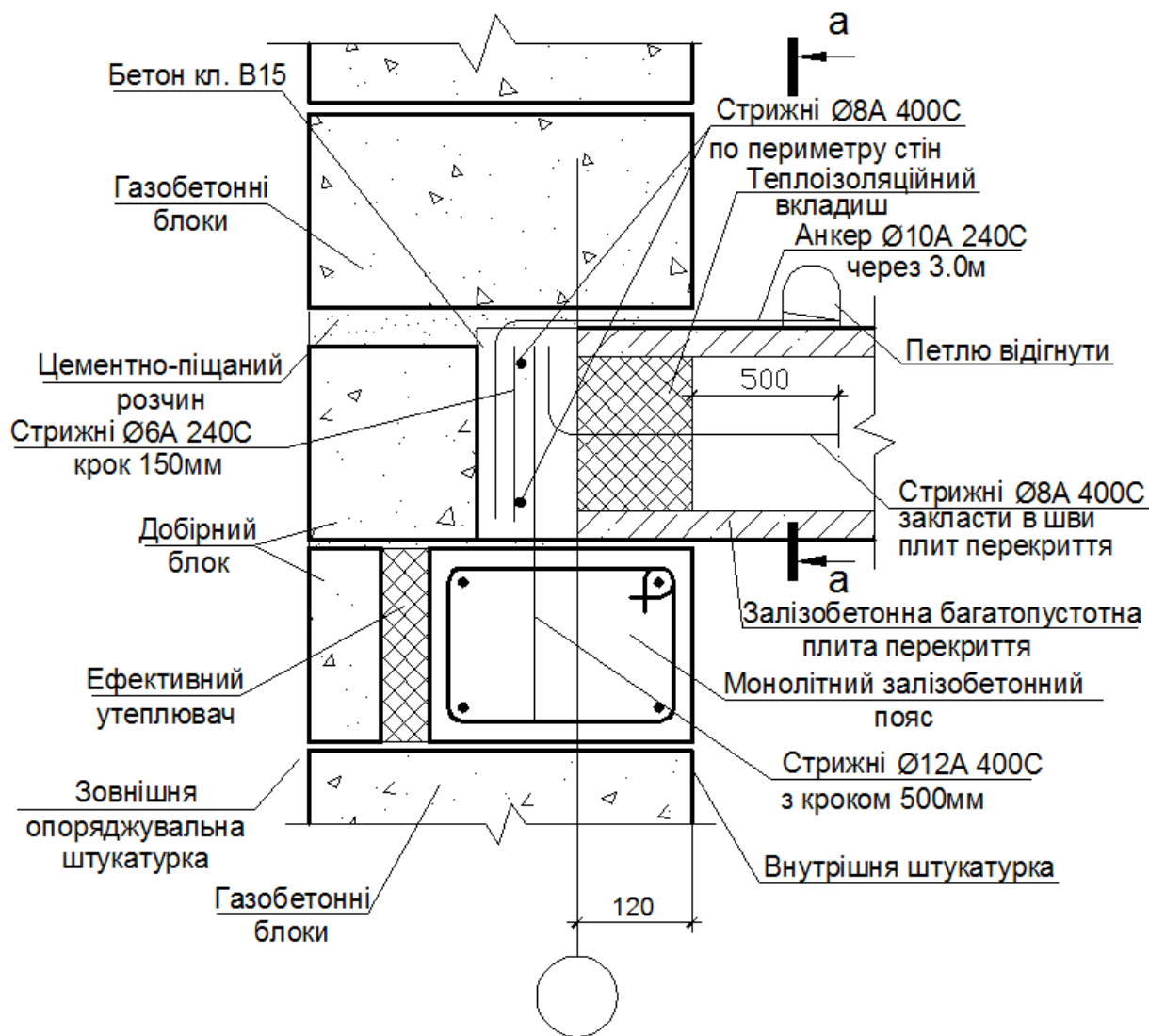
Рис. 2.8-6. Спирання збірного залізобетонного перекриття на монолітний пояс
