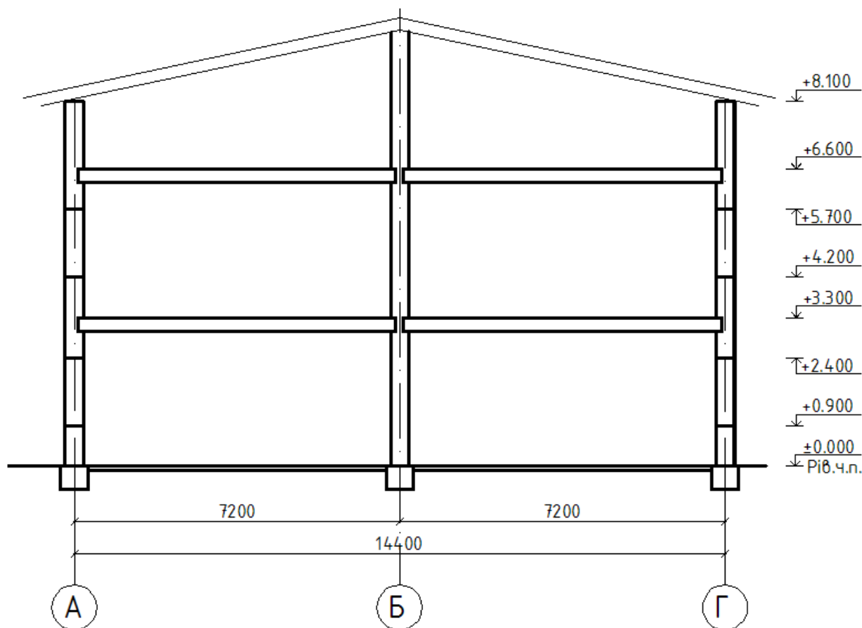
Рис.2.3-2. Поперечний розріз 2-поверхового будинку з мансардою
