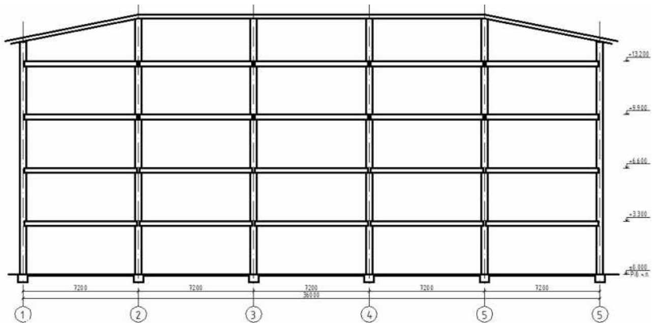
Рис.4.2-2. Повздовжній розріз 4-поверхового будинку
