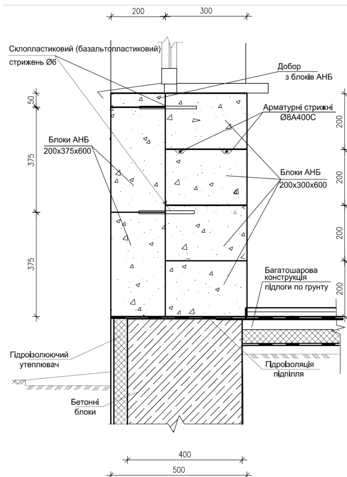
Рис.2-12-2. Двошарова стіна першого типу. Вузол спирання стіни на блок фундаменту
