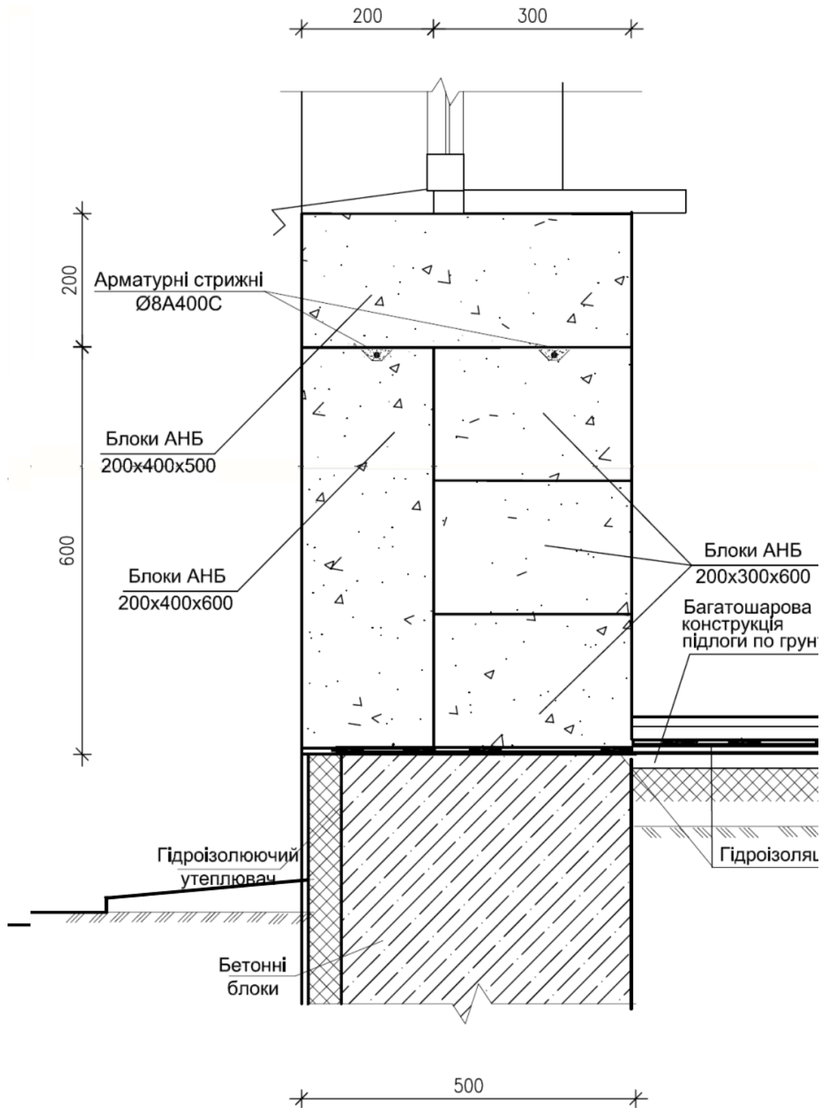
Рис.2-12-9. Двошарова стіна другого типу. Вузол спирания стіни на блок фундаменту.
