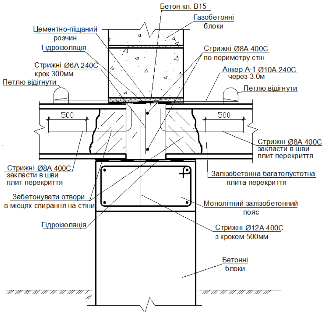
Рисунок 2.2-7. Спирання залізобетонного перекриття на фундамент внутрішньої стіни (для 5 поверхів).
