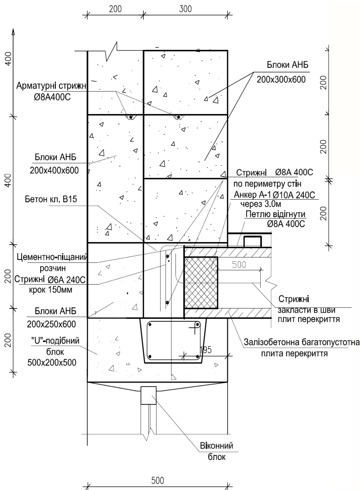
Рис.2-12-7. Двошарова стіна другого типу. Вузол спирання плити перекриття. Висока перетинка (над вікном)
