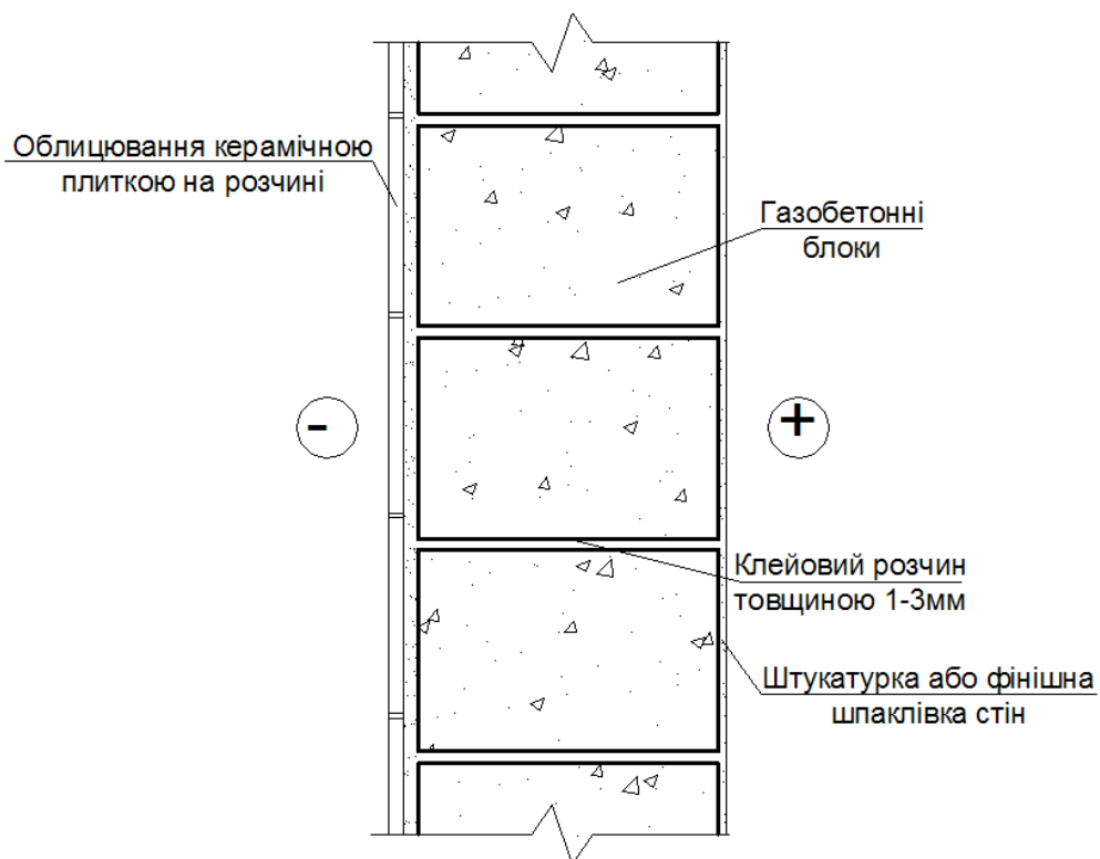
Рисунок 1. 7-2. Стіна з опорядженням личкувальною плиткою
