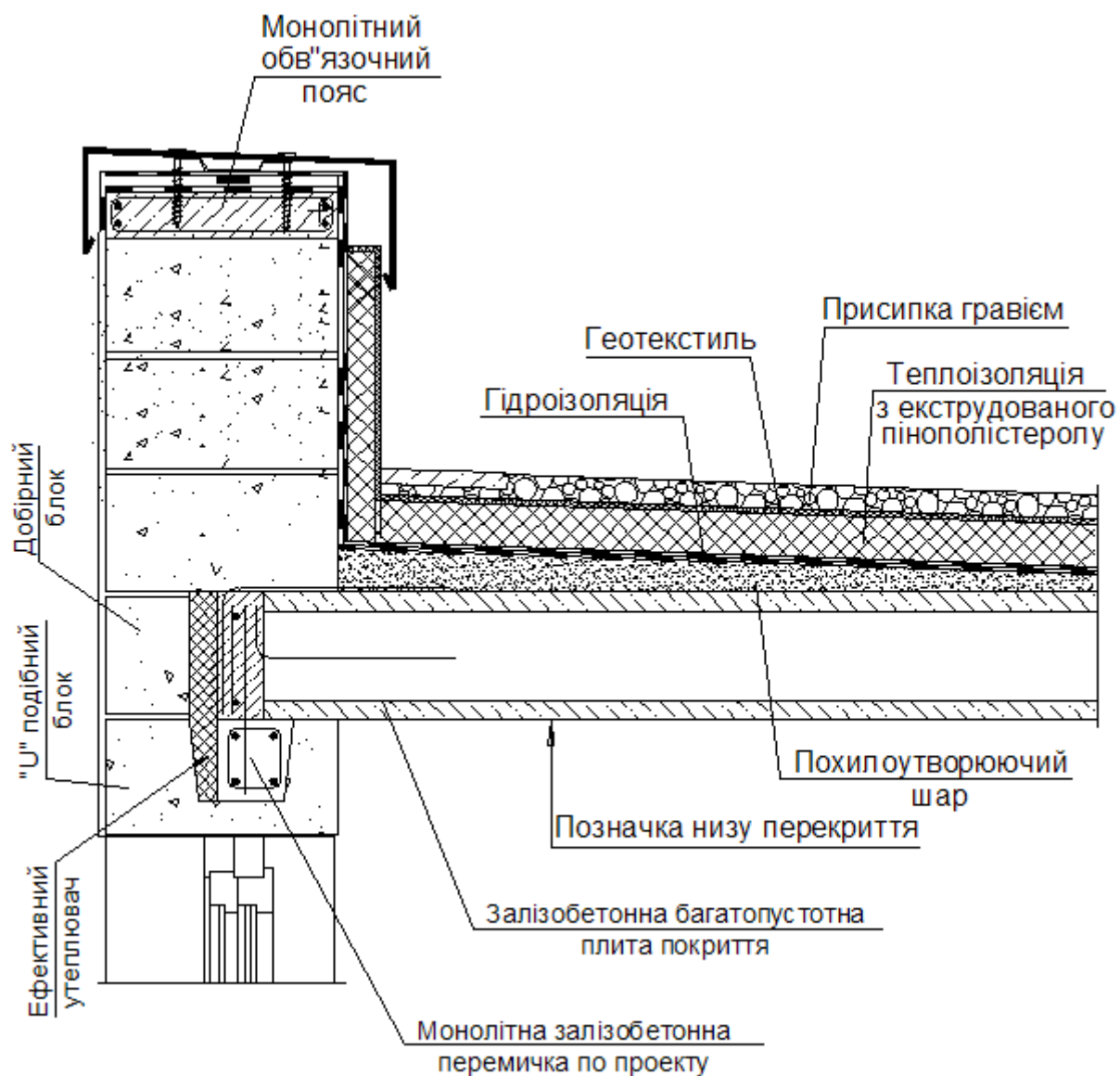
Рис.2.9-8 Конструювання утепленого плаского даху над збірним багатопорожнистим перекриттям даху (варіант з високим парапетом) Проекція здовж пустот
