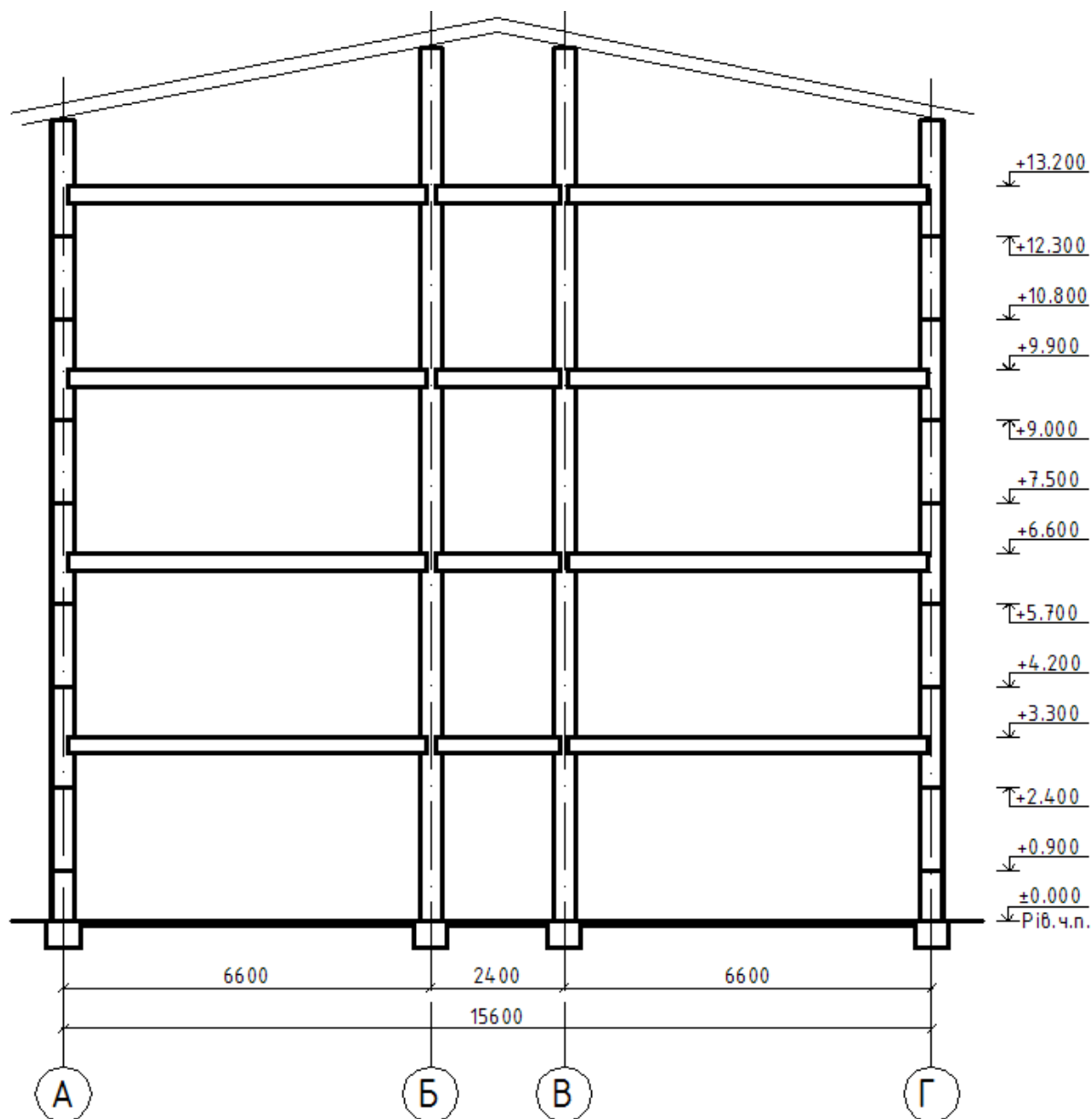
Рис.4.2-3. Поперечний розріз 4-поверхового будинку з мансардою
