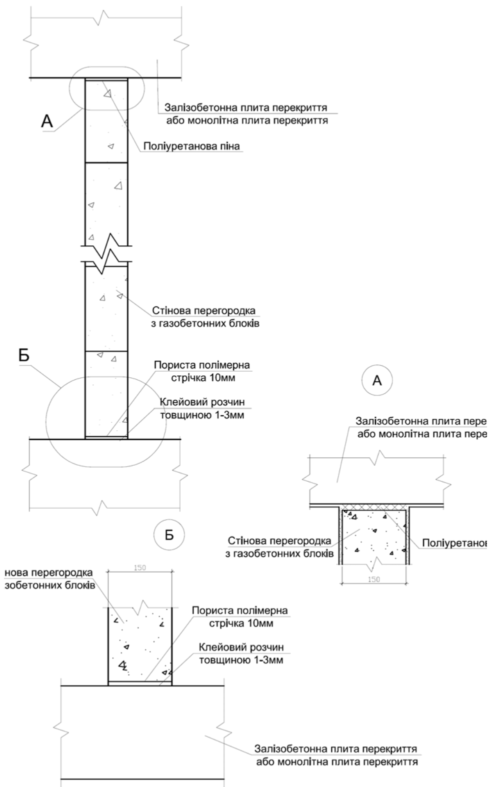
Рисунок 2.2-3. Варіанти примикання перегородок до стін
