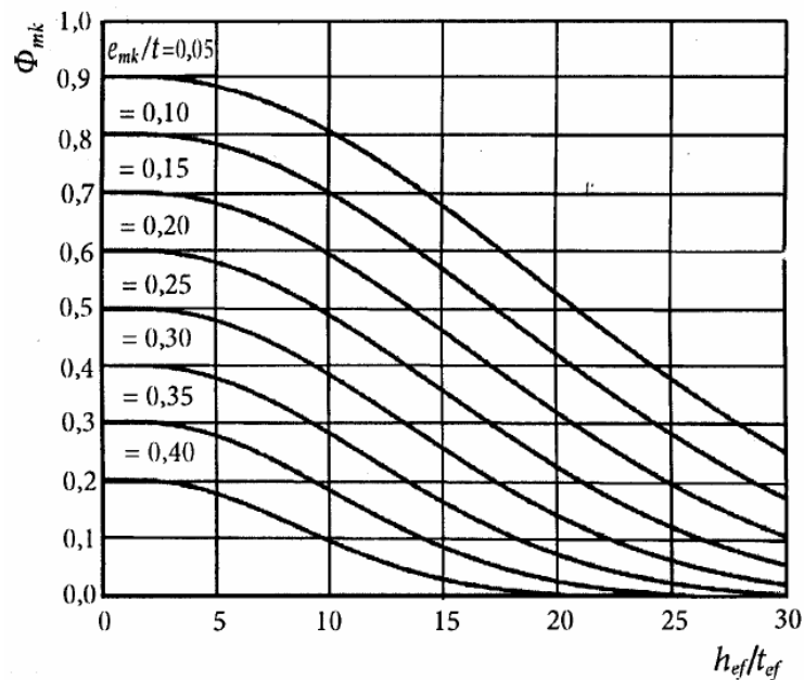
Рис. 1.5-2. Графіки модулів пружності за ДБН В.2.6-162.
