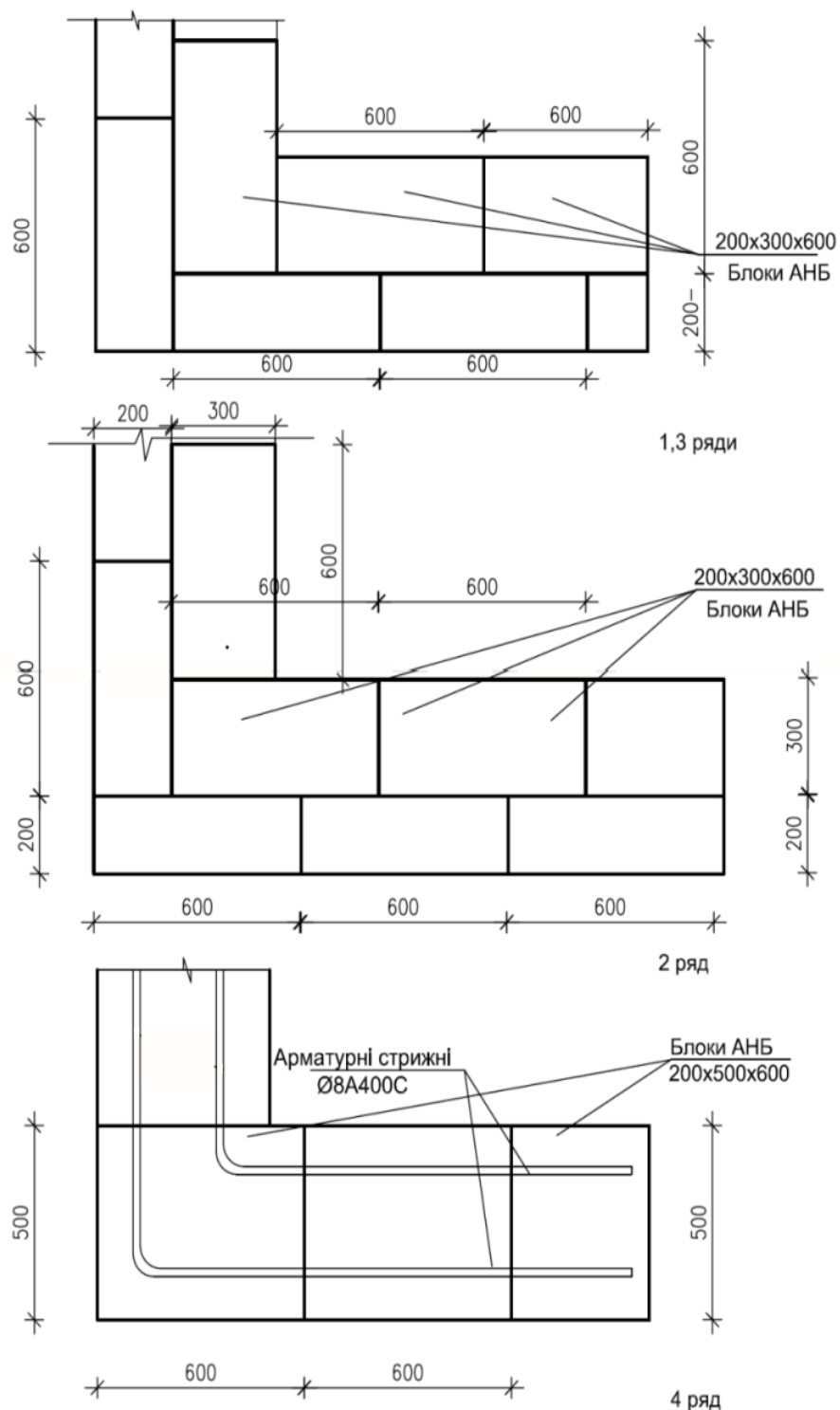
Рис.2-12-11. Двошарова стіна другого типу. Варіант кутової кладки з перев'язуванням і армуванням
