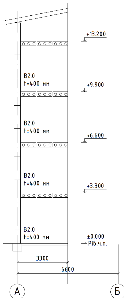
Рис.4.2-8. Матеріали і товщини зовнішньої стіни за результатами розрахунку
