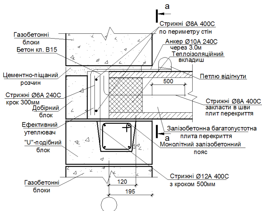
Рисунок 2.1-2. Принципова схема прив'язки стіни до осі
