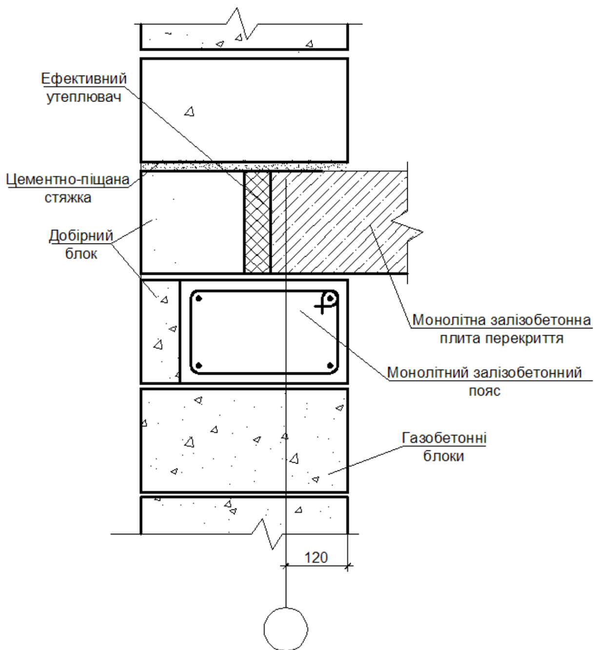
Рис. 2.8-4. Спирання монолітного залізобетонного перекриття на монолітний пояс при прогонах 7,2 м
