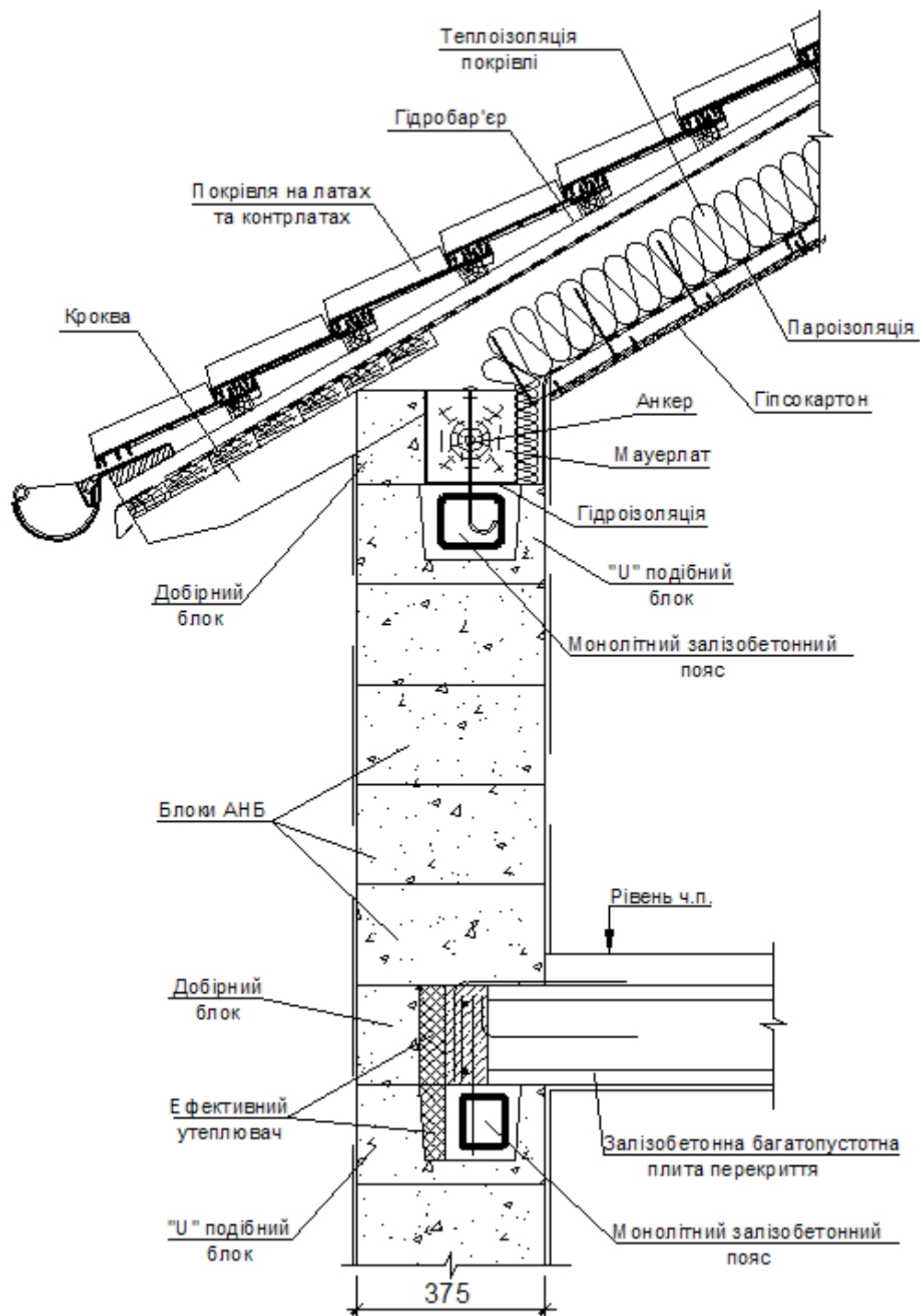
Рис.2.9-2. Конструювання утепленого скатного даху
