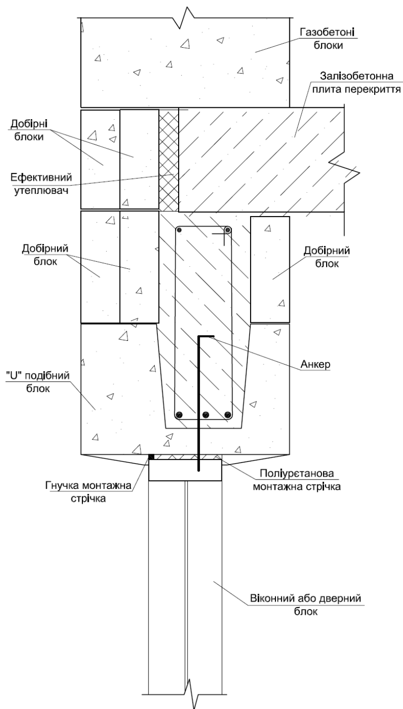
Рис.2.11-5. Схема анкерування воріт
