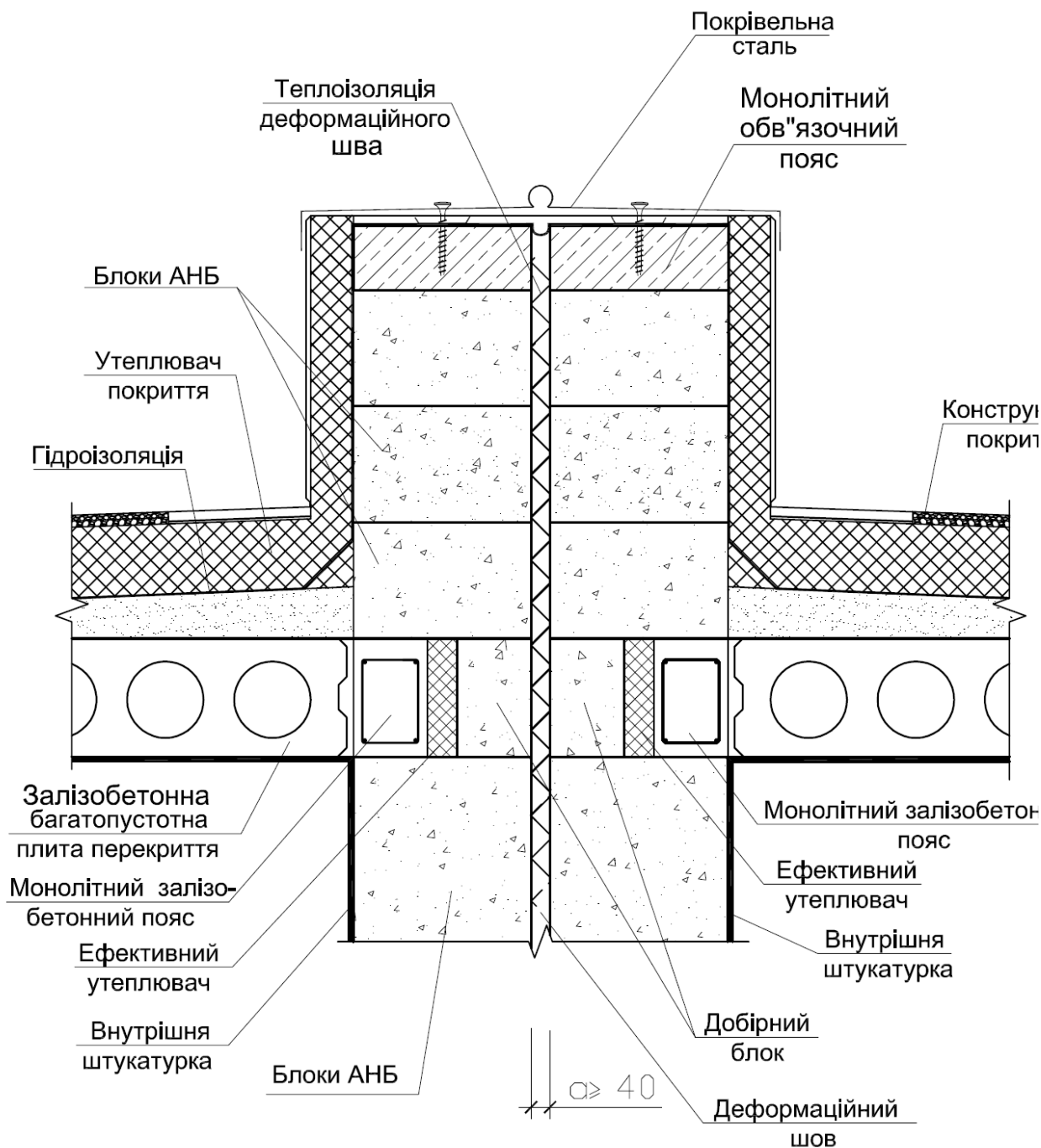
Рис. 3.3. Деформаційний шов у блокованому або секційному будинку з високим вінцем. Покриття - багатопорожнисті плити
