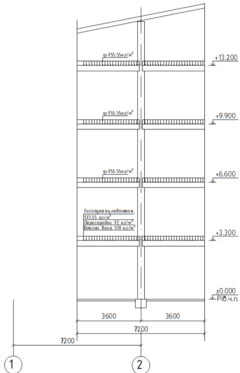
Рис.4.2-6. Навантаження середньої стіни
