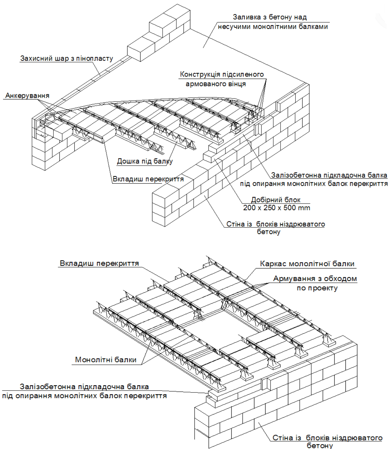
Рис.2.8-1. Дрібноштучне збірно-монолітне перекриття на основі вкладишів з блоків АНБ загальна схема конструювання (зверху) створення наскрізних отворів в перекритті (знизу)
