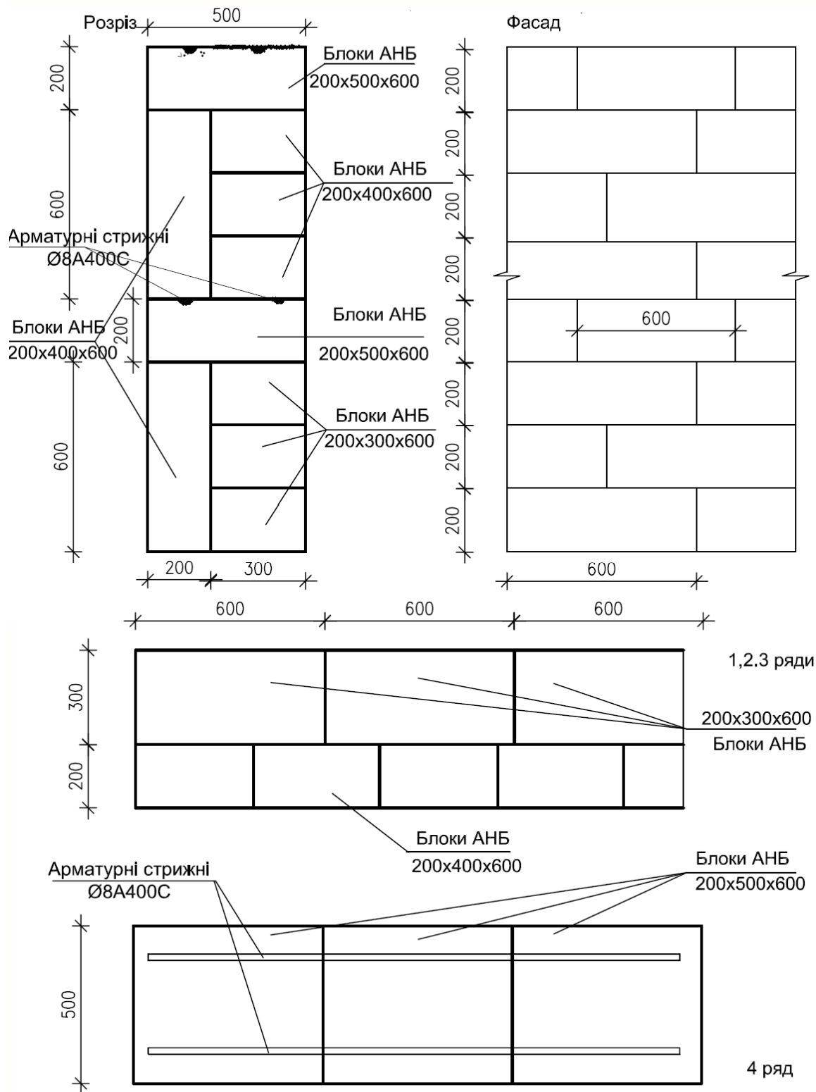
Рис.2-12-10. Двошарова стіна другого типу.
