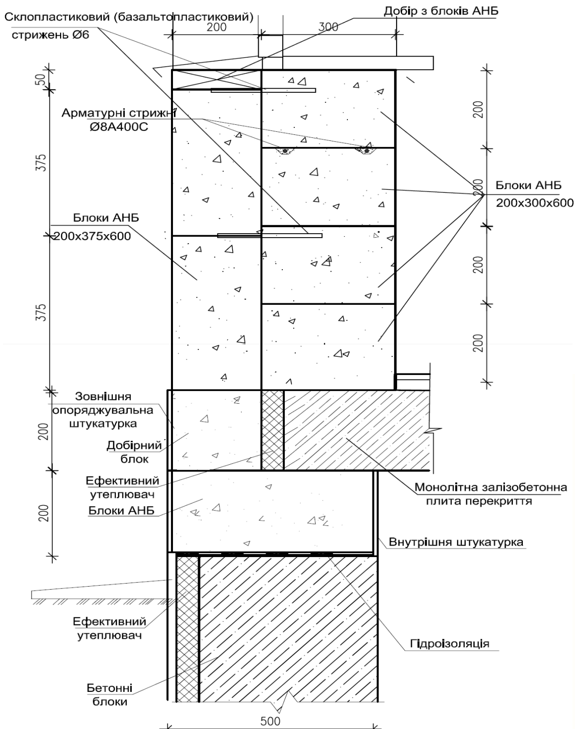
Рис.2-12-3. Двошарова стіна першого типу. Вузол спирання стіни на блок фундаменту. Варіант з підвалом і монолітним перекриттям
