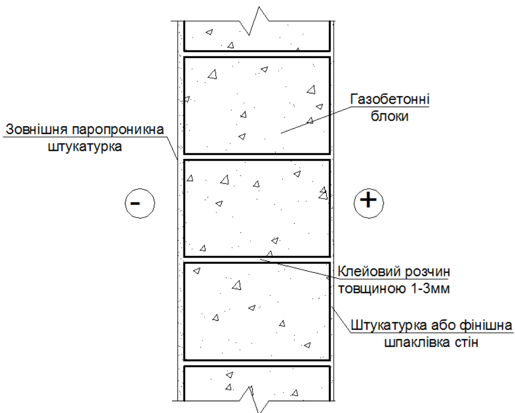
Рисунок 1. 7-1. Одношарова стіна
