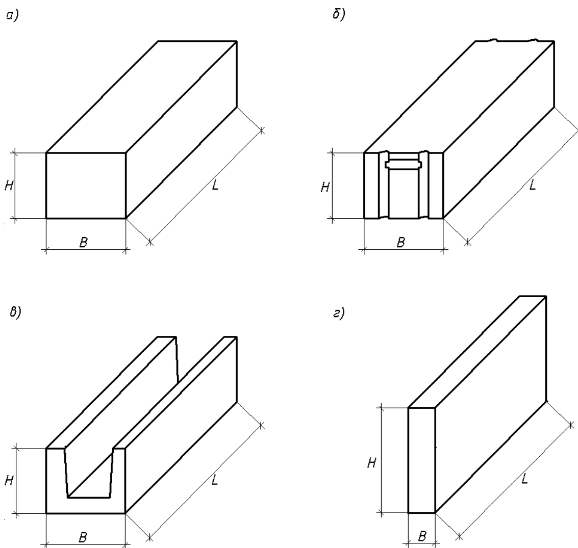
Рис. 1.1. Номенклатура блоків і плит ніздрюватого бетону
