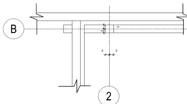
Рисунок 5.1-2. Сільськогосподарська споруда (сховище овочів). Стіни у створі колон. Проект розроблено в ДП «УкрНДІпроцивільсьбуд»
