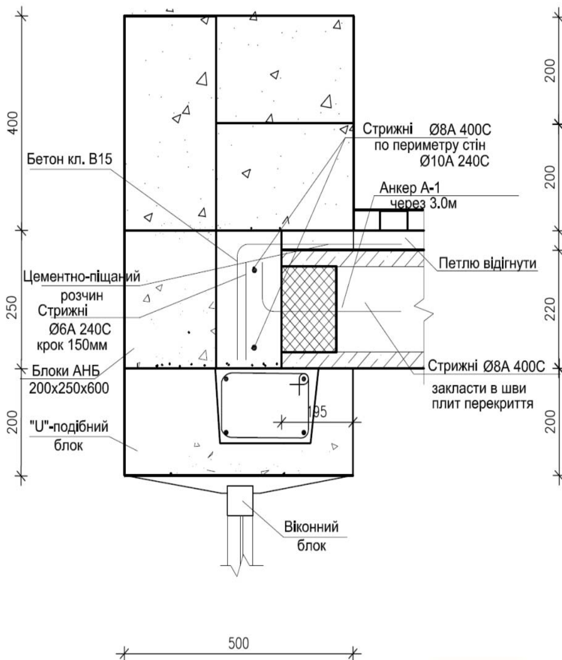
Рис.2-12-16. Двошарова стіна третього типу. Вузол спирання плити. Висока перемичка або монолітний пояс під спирання
