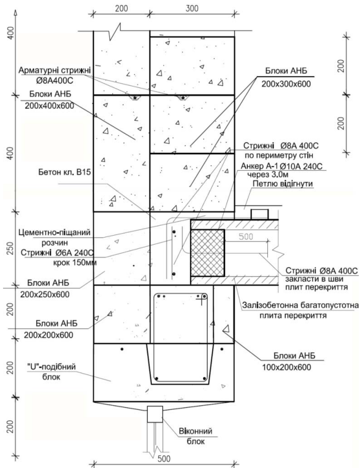
Рис.2-12-6. Двошарова стіна другого типу. Вузол спирання плити перекриття. Перетинка над великим отвором
