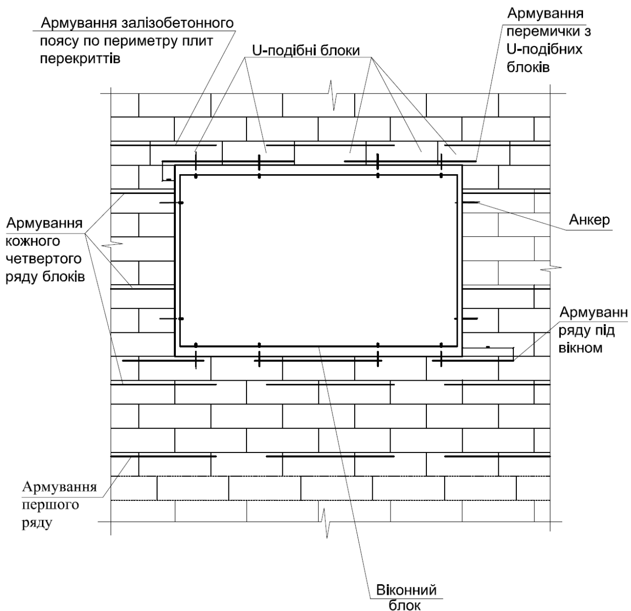
Рис.2.11-1. Схема анкерування вікон у отворах
