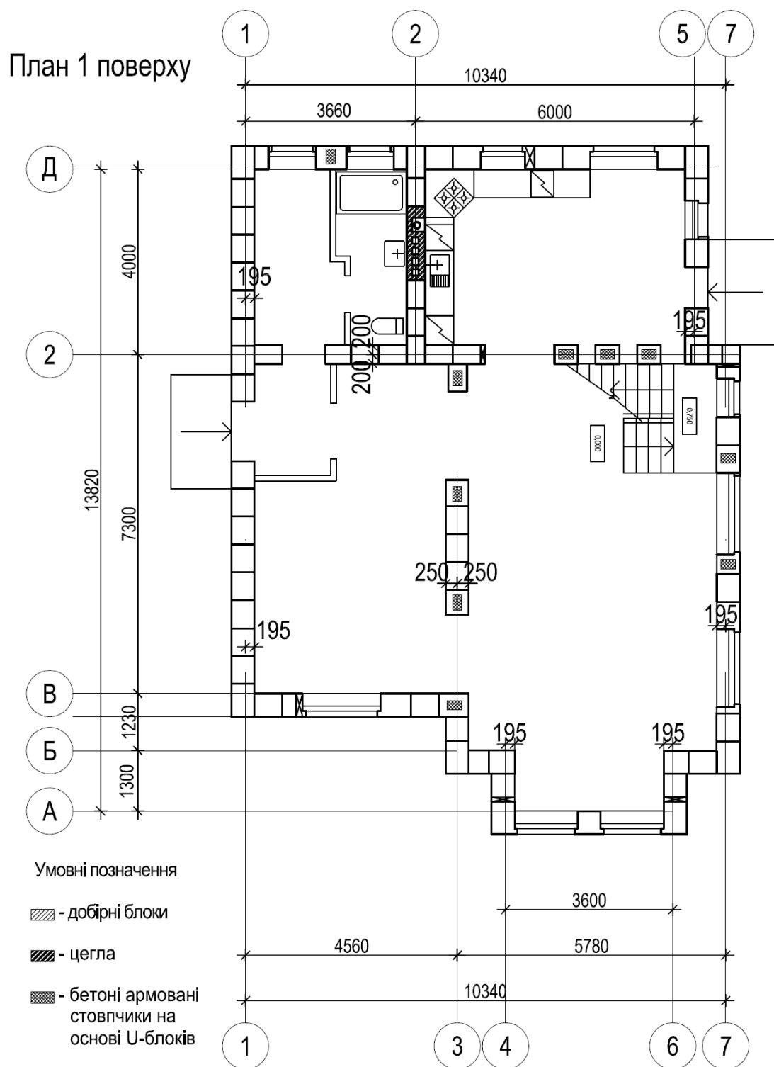
Рисунок 2.1-1. Розбивання вісей на моделювання стін з блоків АНБ в одноквартирному житловому будинку. Проект ДП «УкрНДІпроецивільсільбуд».
