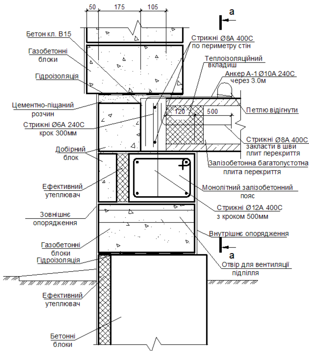
Рисунок 2.2-4. Влаштування цоколя при залізобетонному багатопустотному перекрытті.
