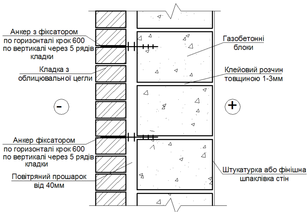
Рисунок 1. 7-3. Двошарова стіна з облицюванням цеглою і повітряним прошарком
