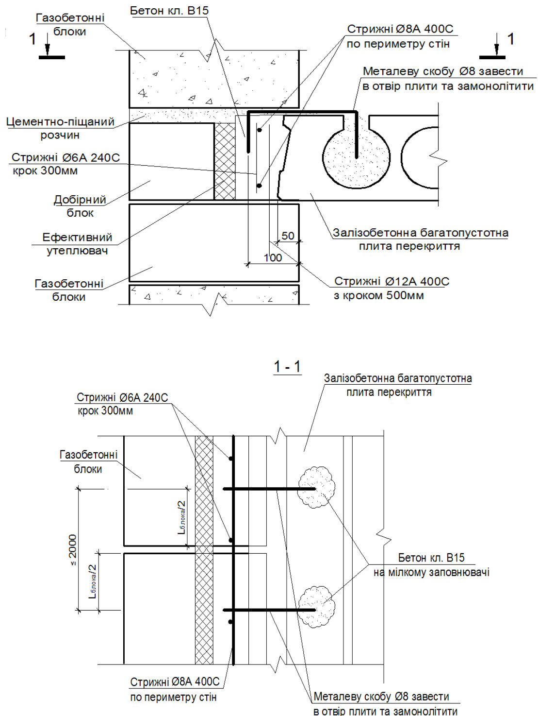
Рис. 2.8-3. Анкерування збірних багатопорожнистих плит перекриття
