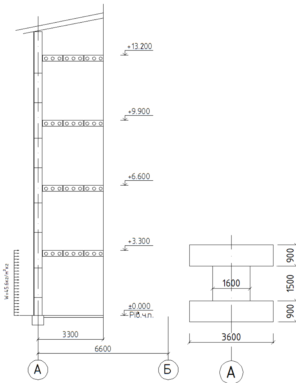
Рис.4.2-4. Схема навантажень простінку зовнішньої стіни
