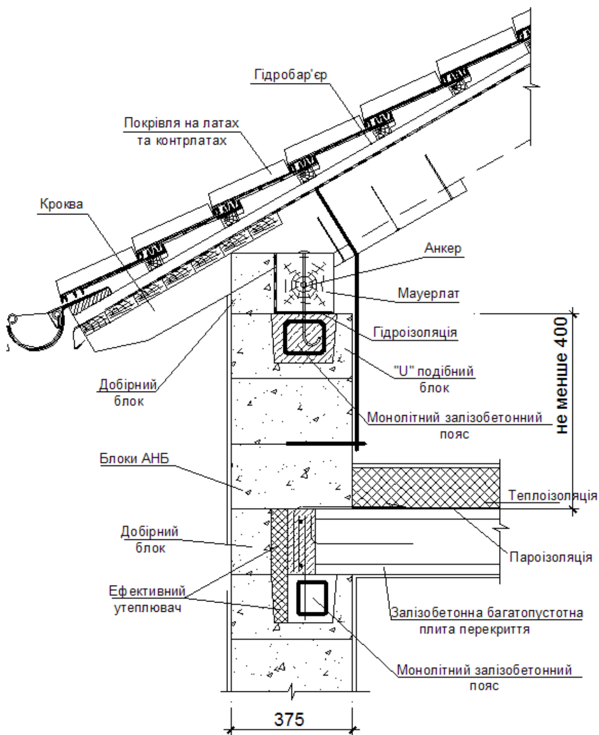
Рис.2.9-1. Конструювання холодного скатного даху
