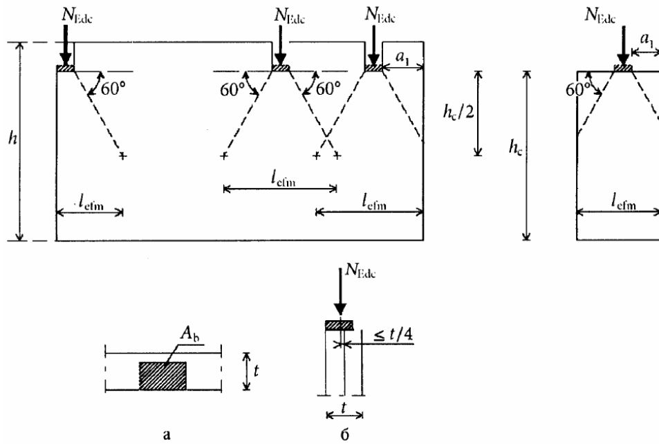
Рис. 1.5-4. Стіни при зосереджених навантаженнях.
