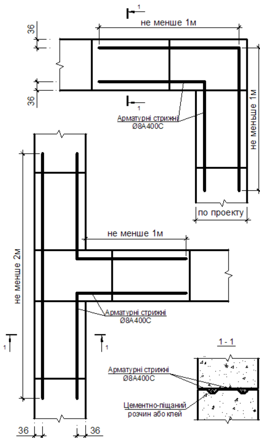
Рисунок 2.7-2. Горизонтальне армування несучих стін
