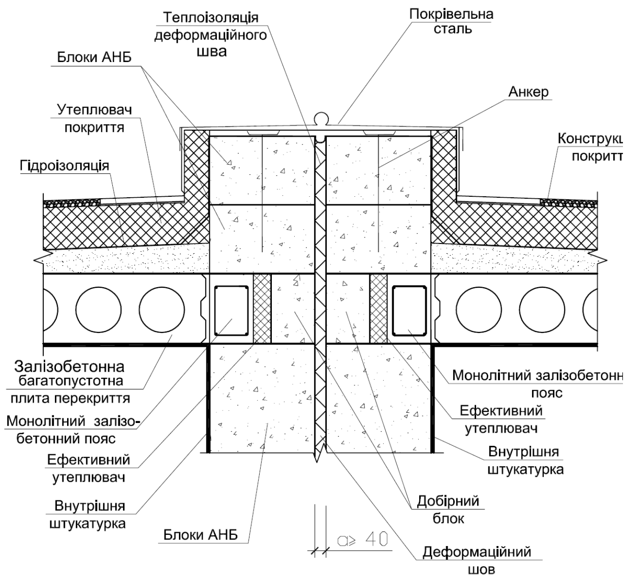
Рис.3.5. Деформаційний шов у блокованому або секційному будинку з низьким вінцем. Покриття - багатопорожнисті плити
