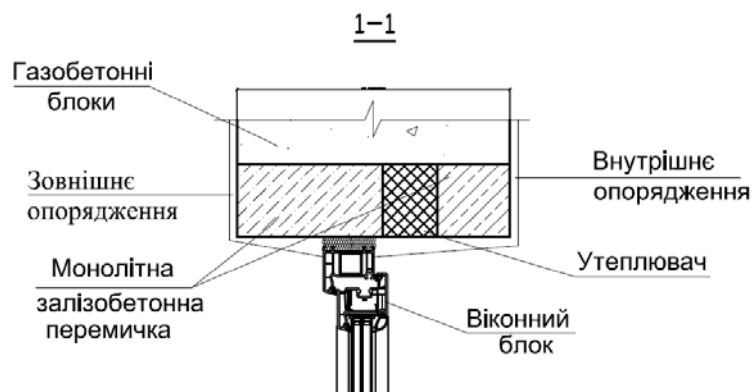
Варіант 3 - Перемичка з монолітного бетону
