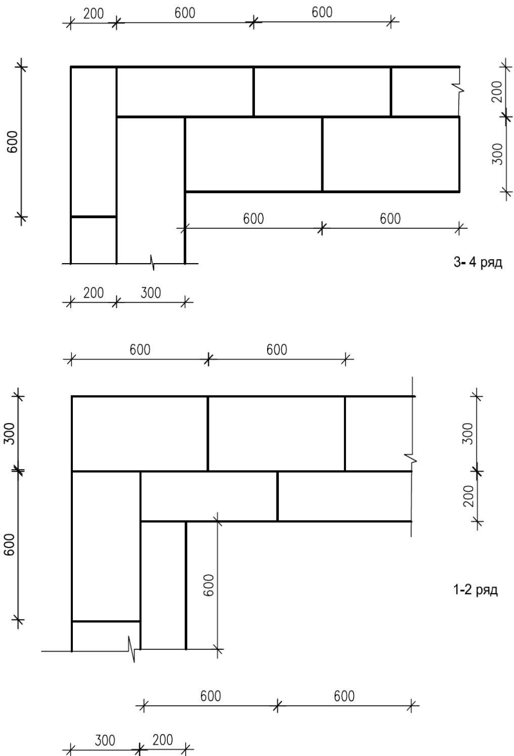
Рис.2-12-15. Двошарова стіна третього типу. Кутове з'єднання
