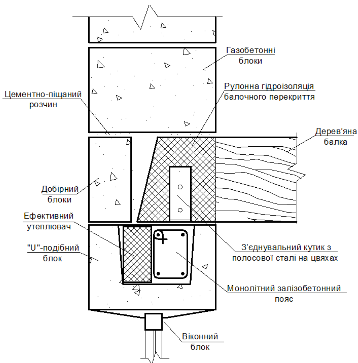
Рис.2.4-2. Перемичка з U-блоків з додатковим ефективним утеплювачем
