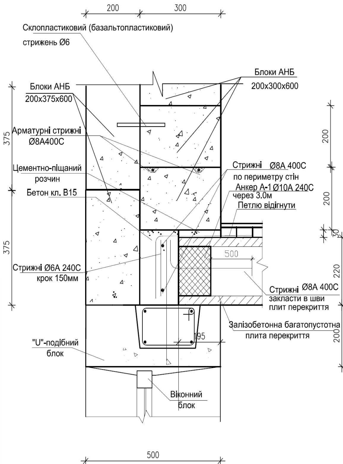
Рис.2-12-1. Двошарова стіна першого типу. Вузол спирання плити перекриття
