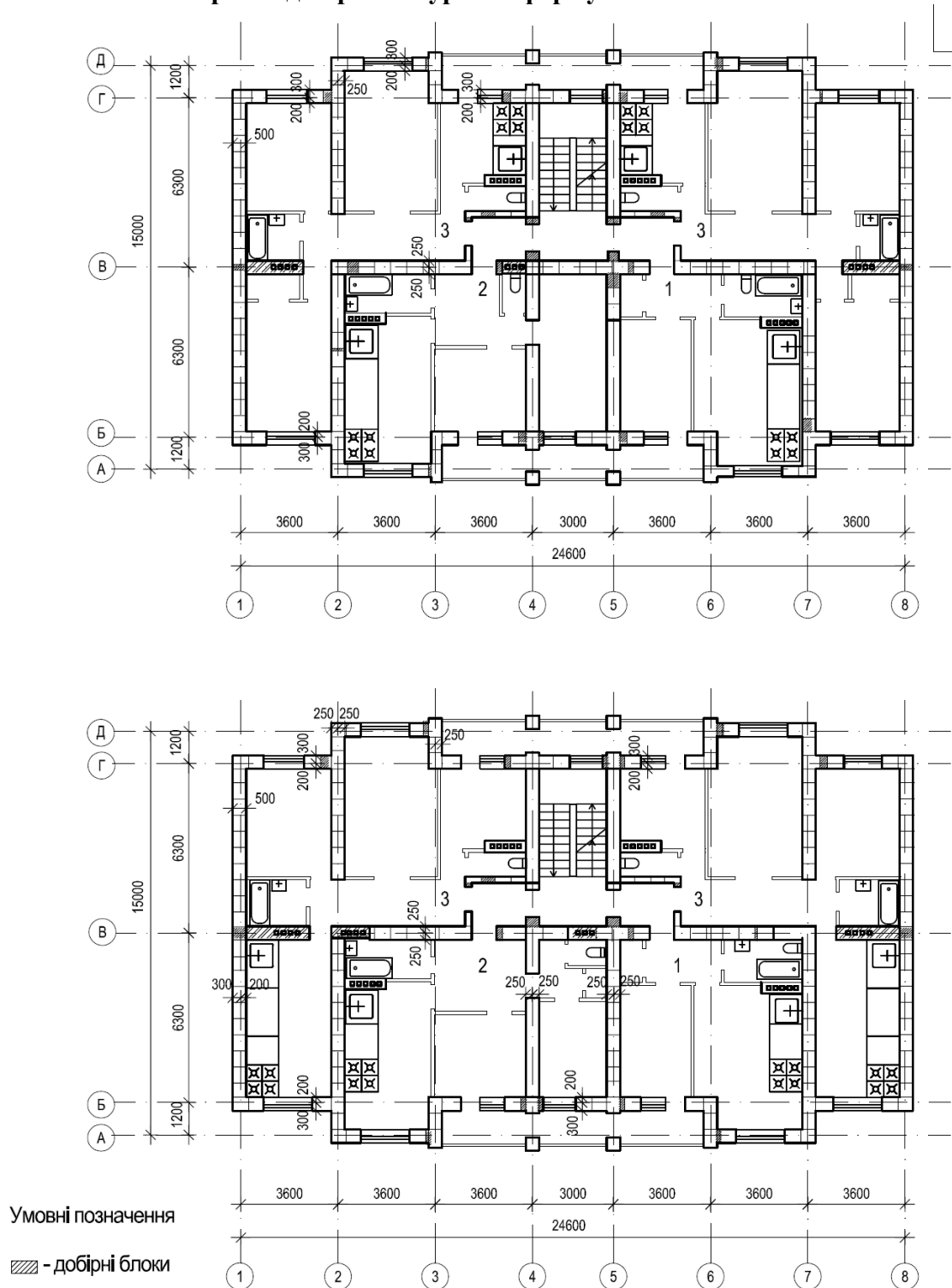
Рис.4.1-1. Широтна 4 –поверхова блок-секція 1-2-3-3 із поперечним кроком несучих стін
