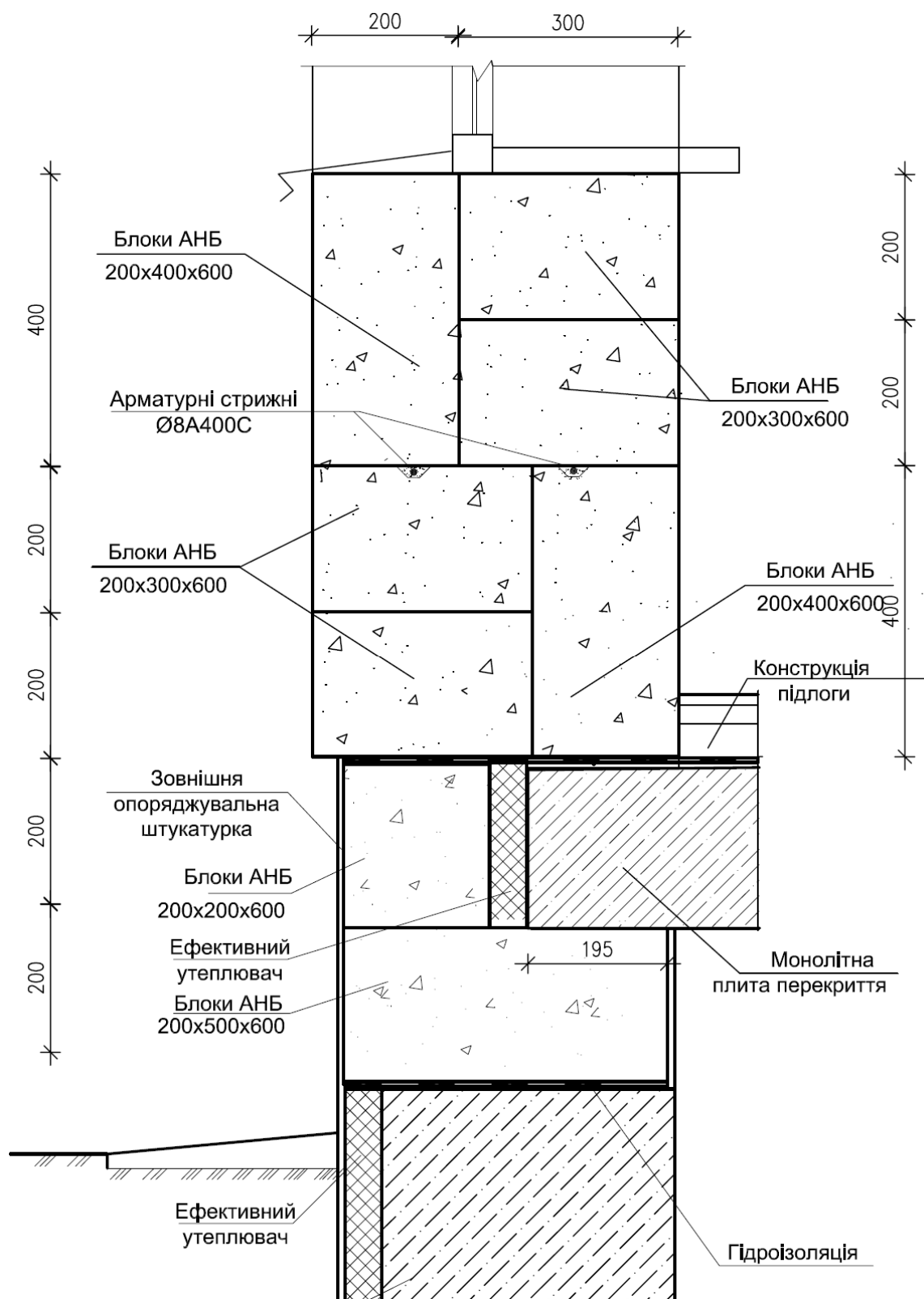
Рис.2-12-13. Двошарова стіна третього типу. Вузол спирання стіни на блок фундаменту. Варіант з підвалом
