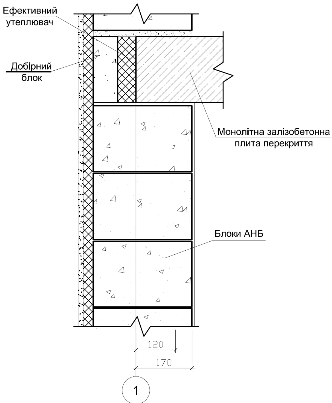
Рис.2.8-3. Спирання монолітного залізобетонного перекриття на зовнішню стіну з АНБ
