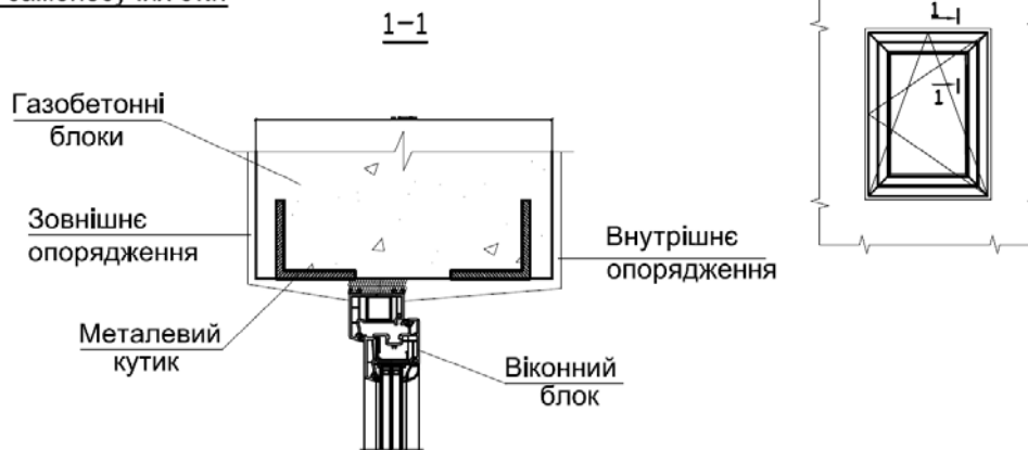
Варіант 1 - Перемичка з металевих кутиків для самонесучих стін
