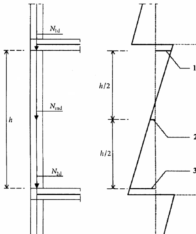
Рис. 1.5-1. Моменти внаслідок ексцентриситету
